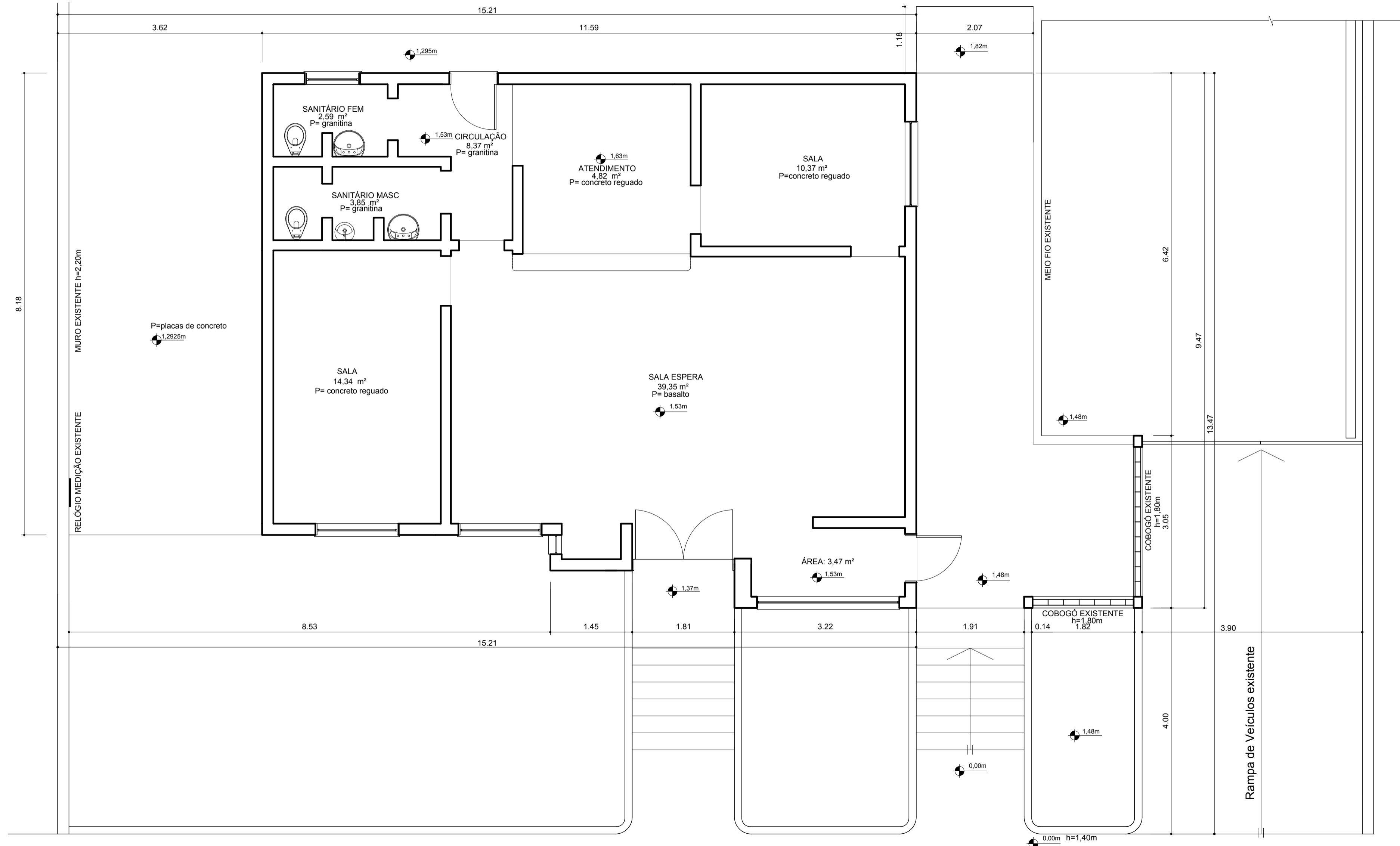
PLANTA BAIXA ATUAL ESCALA: 1/50
